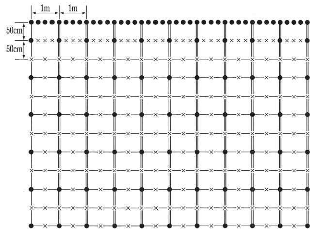
アンカー打設図
