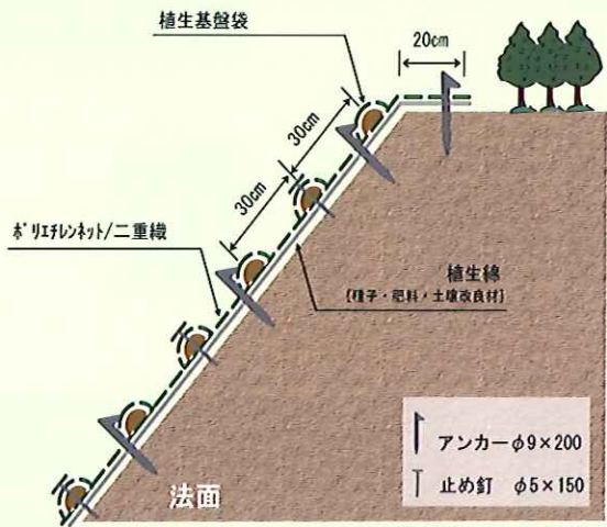
(図は3号I型 植生基盤袋間隔30cm)
