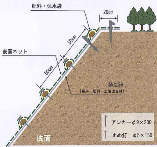
(図はP-50 肥料・保水袋間隔50cm)
