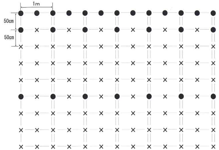
●…アンカーφ9×200 ×…止め釘 φ5×150
